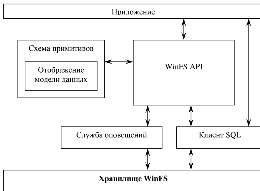
Рис. 3. Архитектура WinFS
