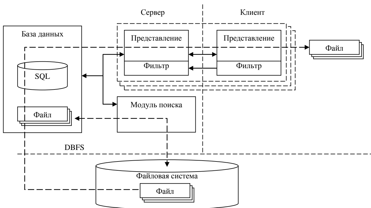
Рис. 4. Представление реализации DBFS
