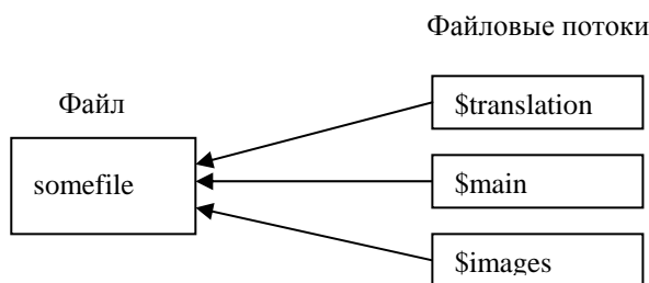
Рис. 2. Файловые потоки
